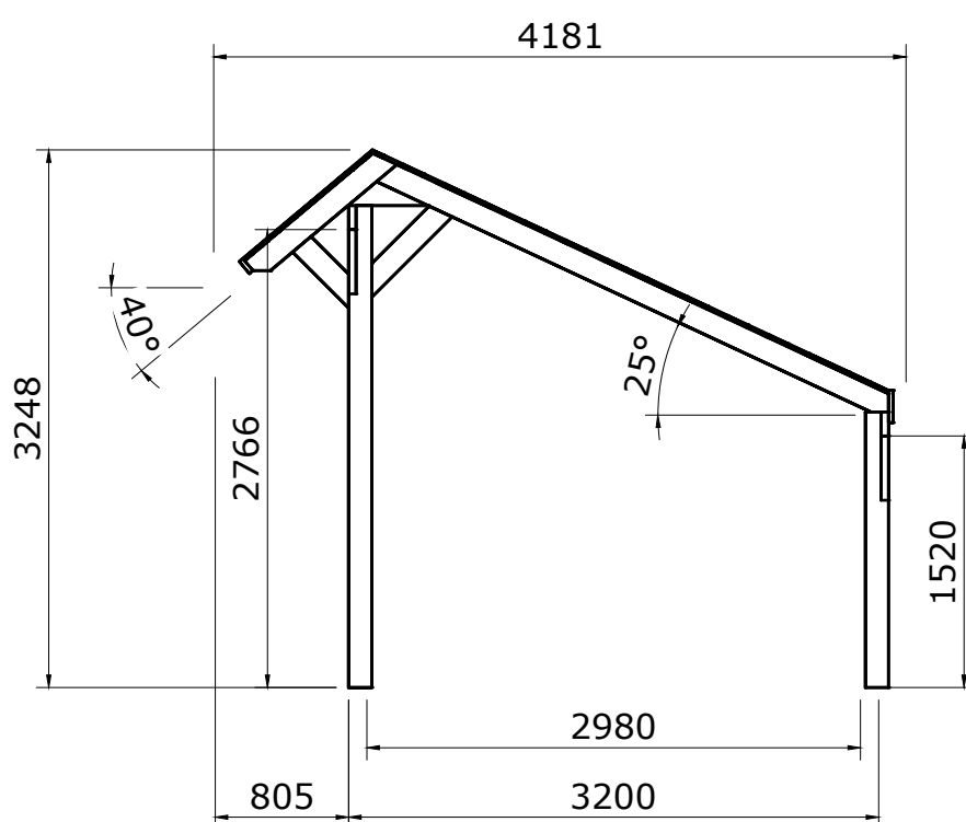
Rechter zijaanzicht
